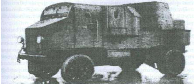
"Garford-Putilovs" zirehli avtomobili. Foto. L.Qoçoqlevin materiallarından
